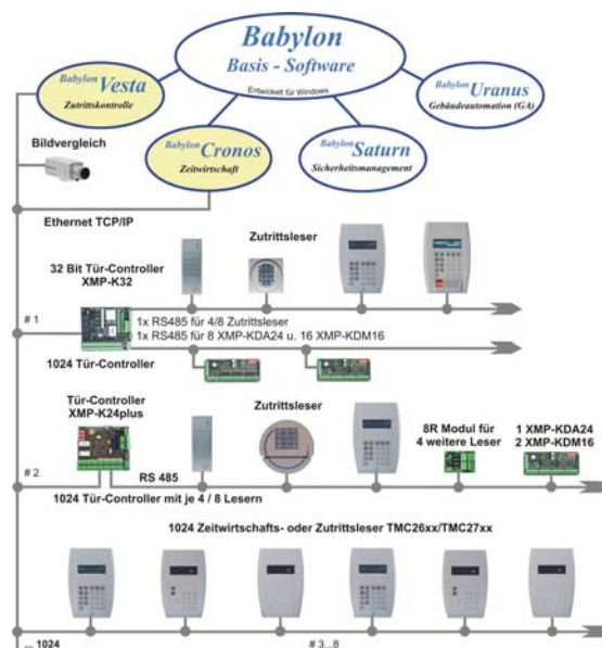
Schema der Anschlussmöglichkeiten für Kartenleser an BABYLON
